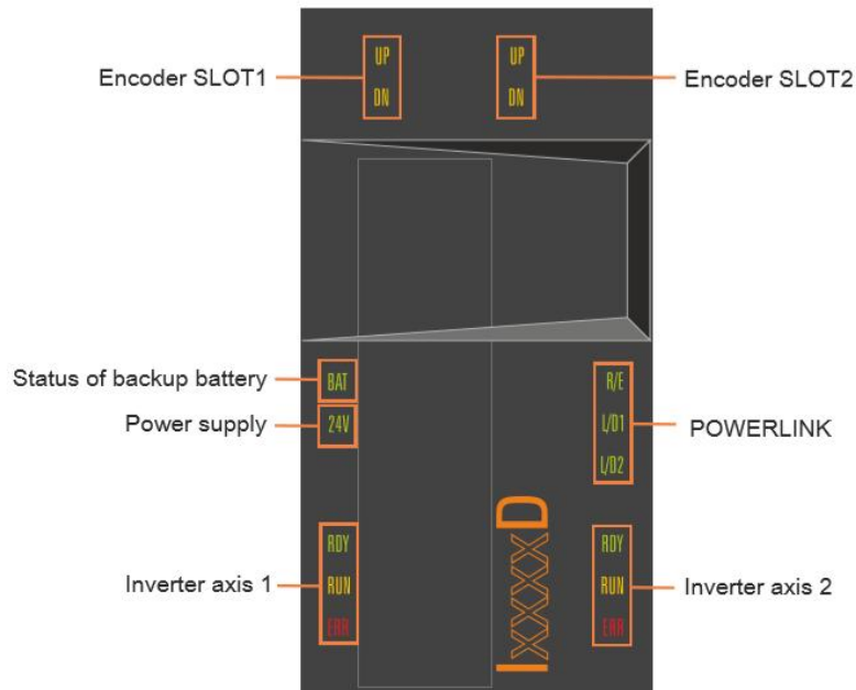
图 3-31 驱动器上 LED 状态指示灯
