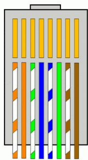
图 2-35 以太网连接
