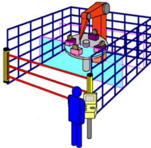
图 2-18 连接安全光幕
