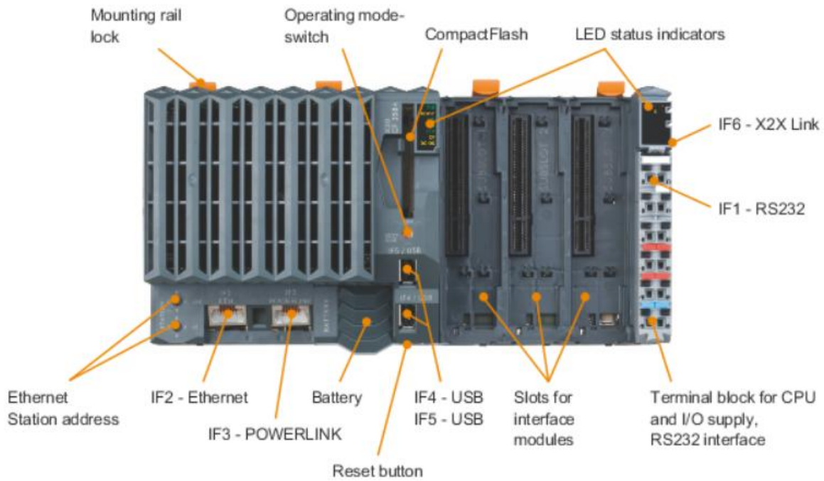
图 3-12 X20CP3584 的组成
