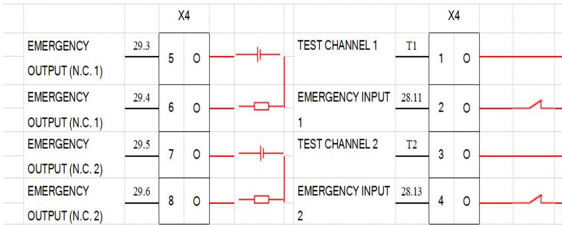
图 2-26 外部急停接线示意图
