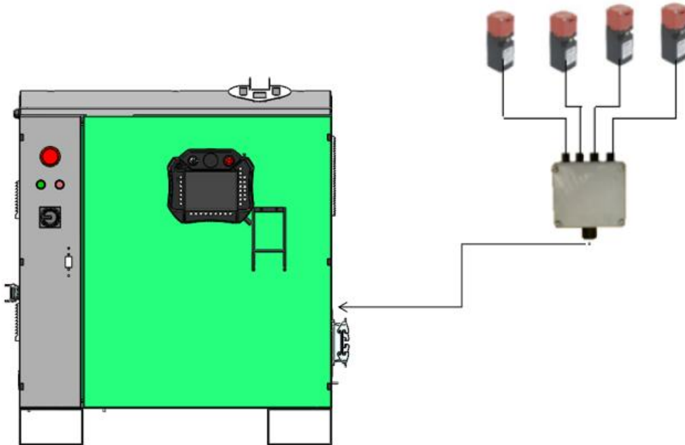
图 2-16 多个安全门连接示意图
