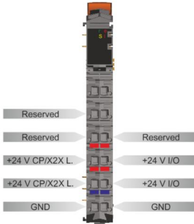
图 3-13 引脚排列
