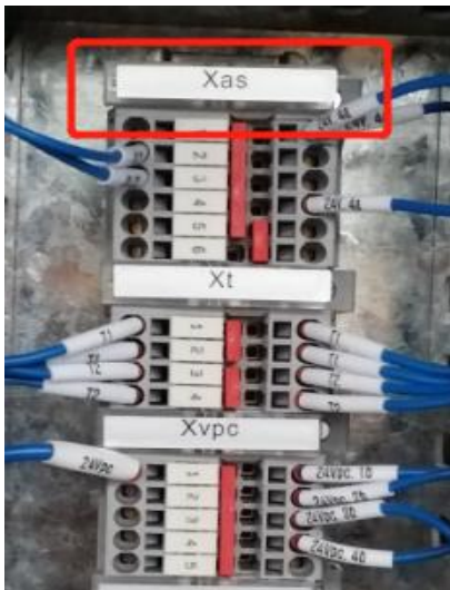
图 2-20 安全光幕的接线
