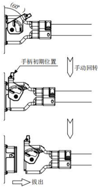
图 2-9 拔出电源线步骤
