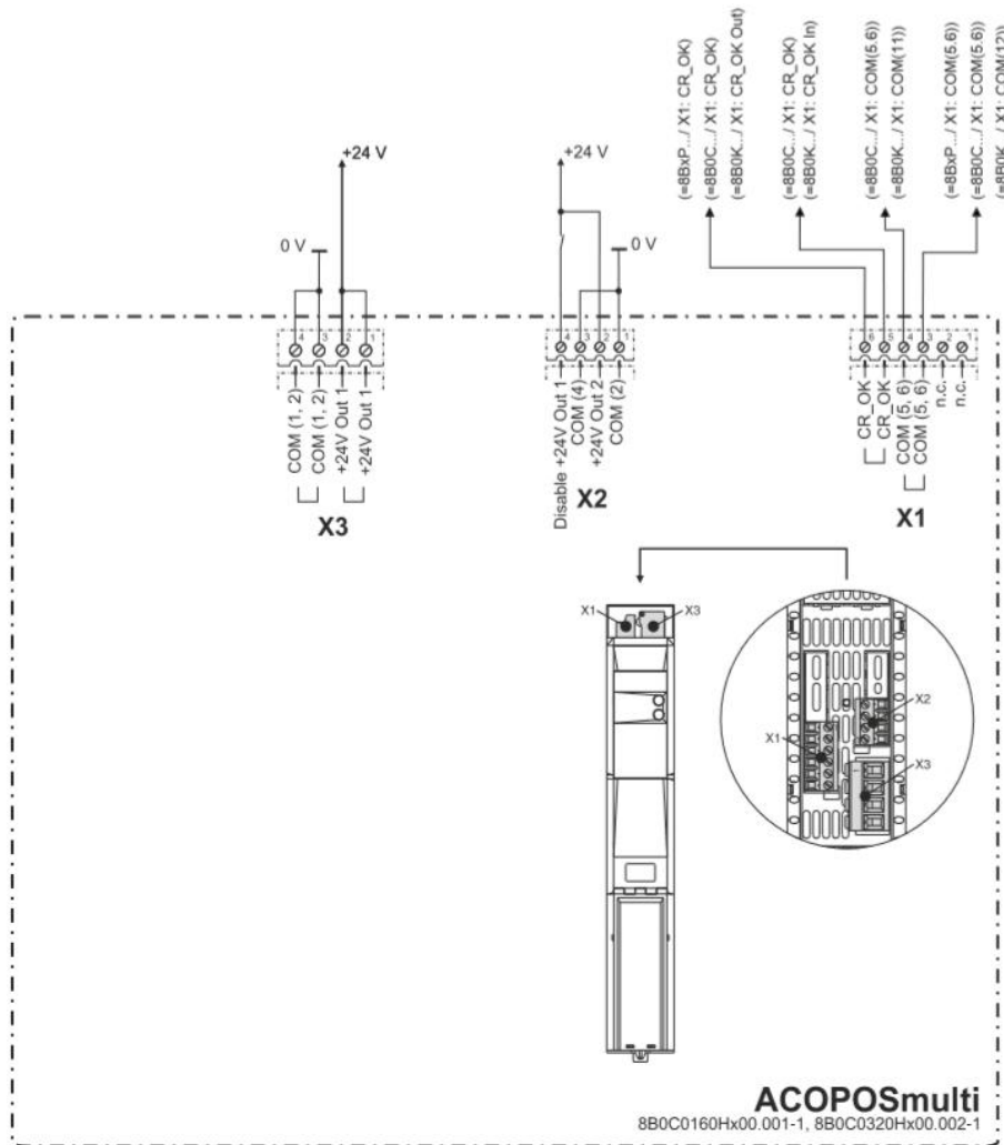
图 3-26 辅助电源模块接线示意图
