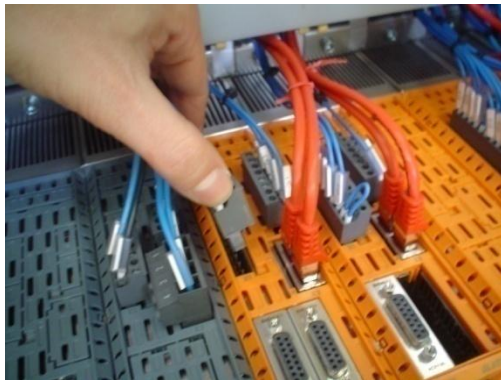
图 4-15 更换驱动器
