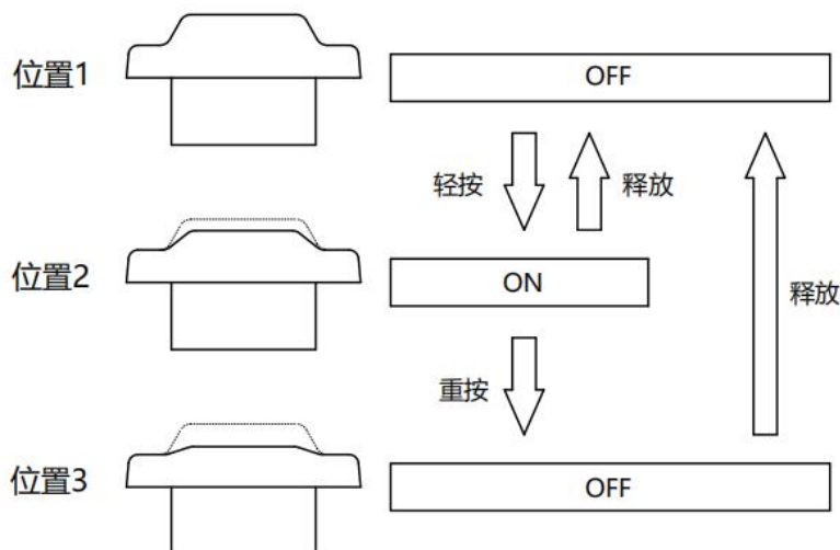
图 3-8 使能开关
