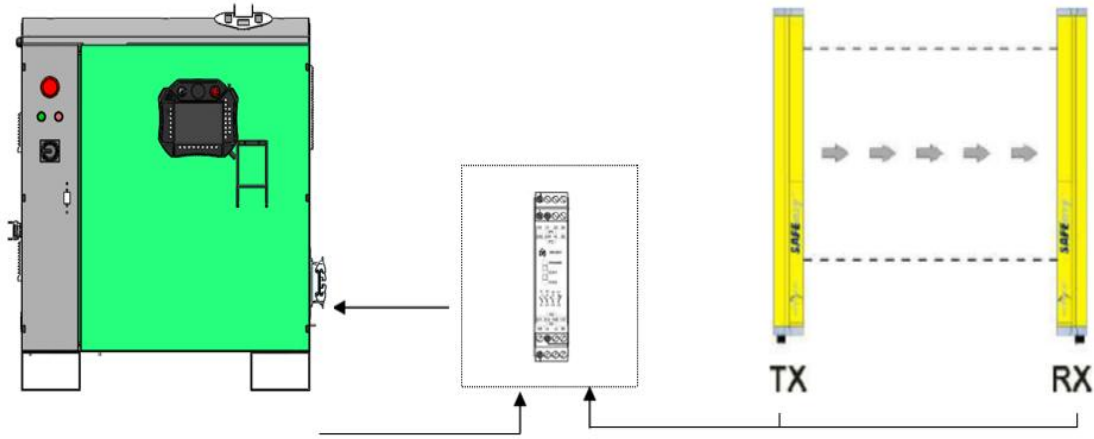
图 2-19 连接安全光幕
