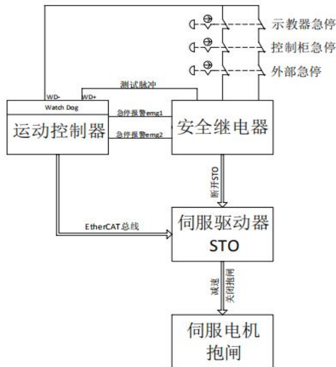
图 3-41 安全功能框图
