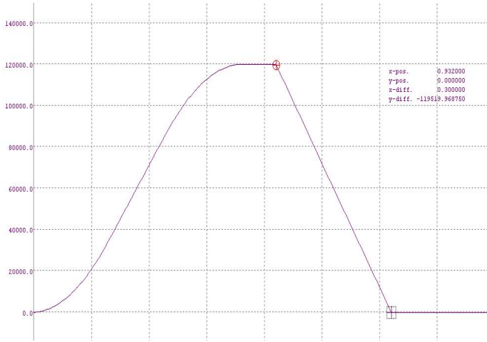
图 2-20 1、2、3 轴停止时间图 选择安全设备, 评估整体安全等级:
