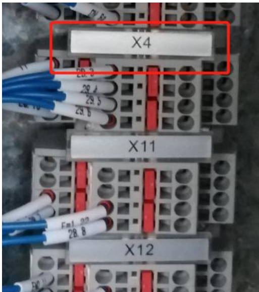
图 2-25 外部急停端子接线
