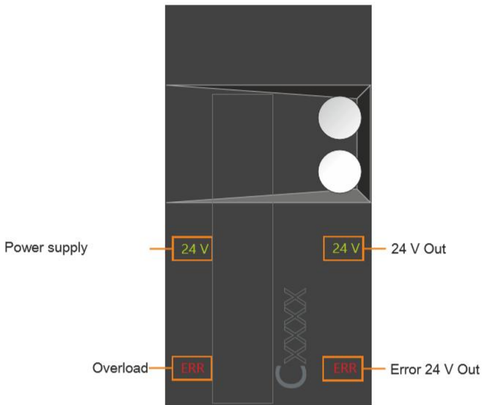
图 3-25 辅助电源模块 LED 状态指示灯
