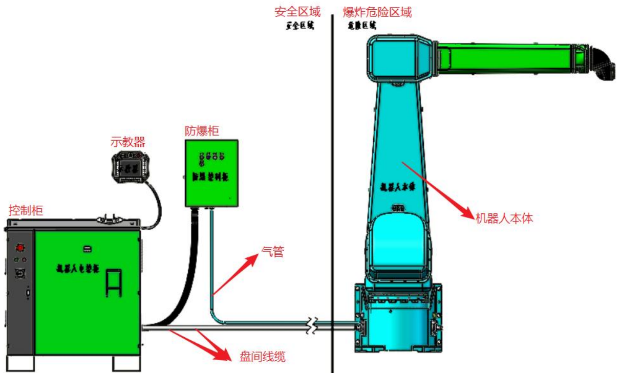
图 2-12 连接机器人
