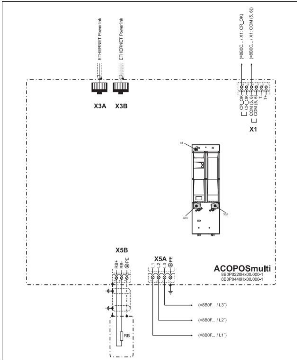
图 3-19 主电源模块接线示意图
