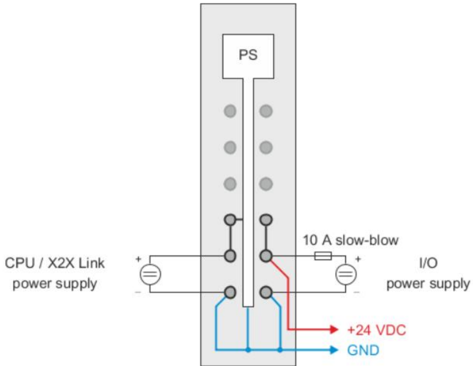
图 3-14 电源连接示意
