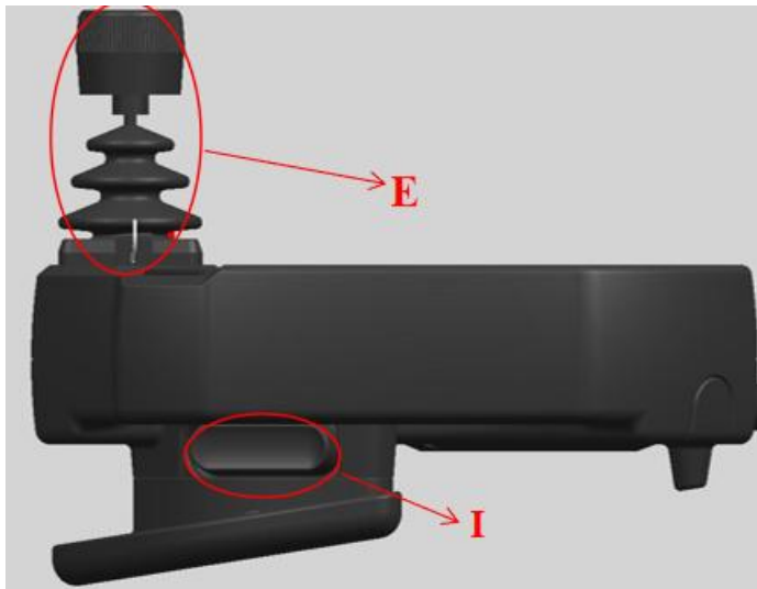
图 3-7 示教器图片
