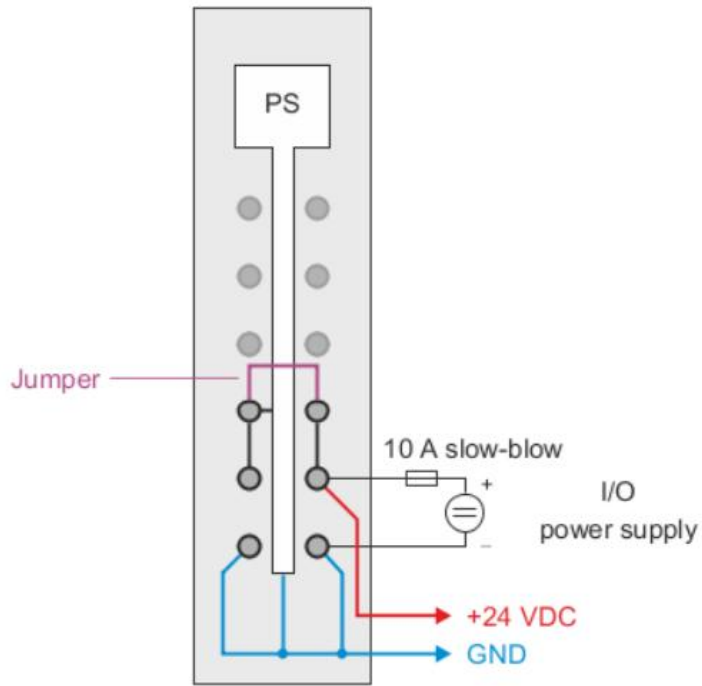
图 3-15 带电源和跳线的连接示例
