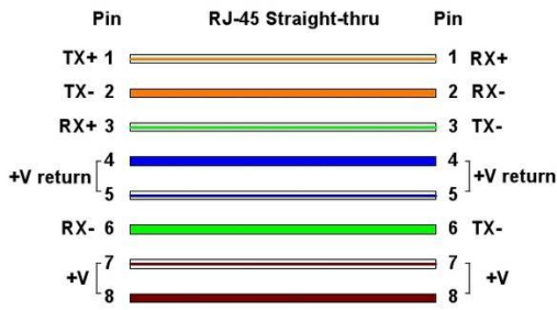
图 2-34 以太网连接
