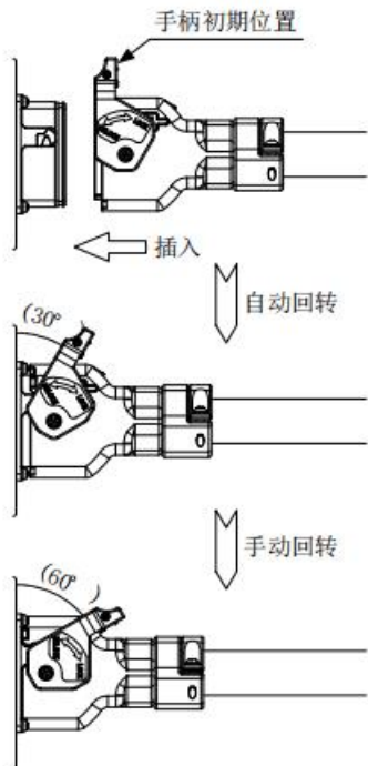
图 2-8 插入电源线步骤
