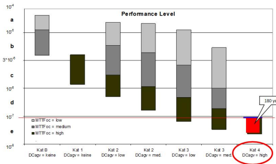
图 2-21 安全等级划分
