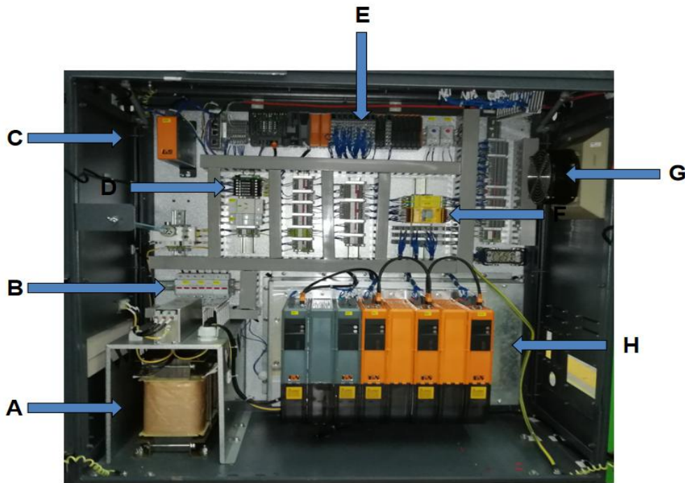
图 3-3 电柜内主要元器件
