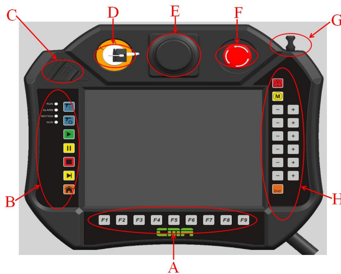
图 3-6 示教器图片
