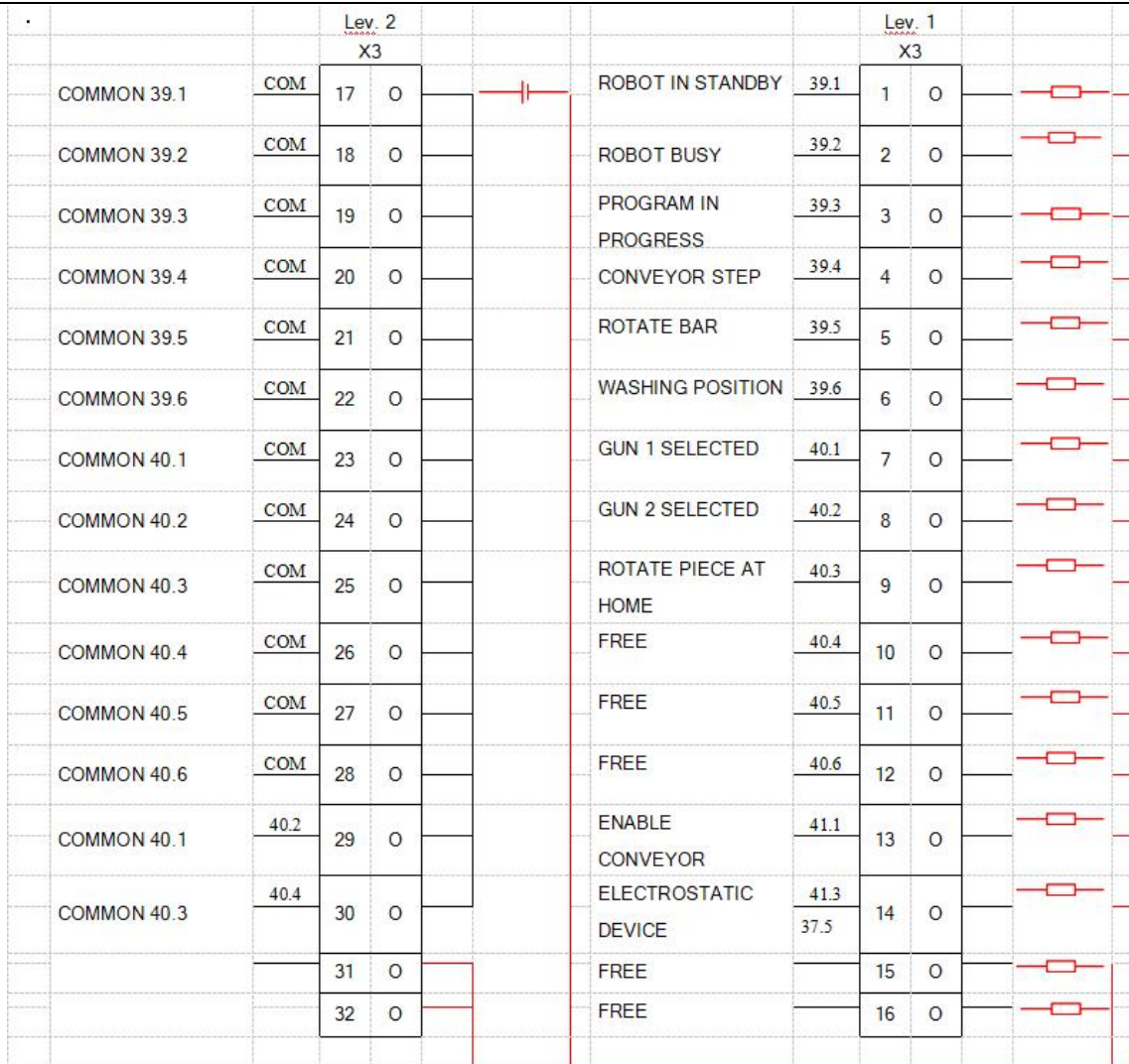
图 2-30 输出信号接线示意图
