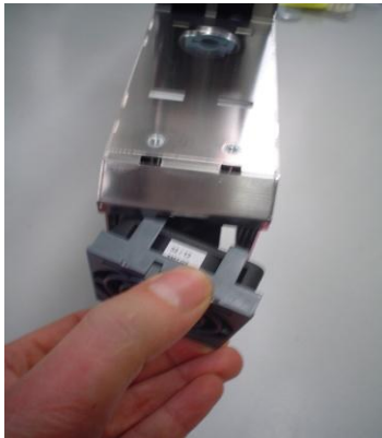
图 4-26 更换驱动器的散热风扇
