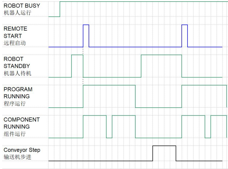
图 2-31 基本时序图
