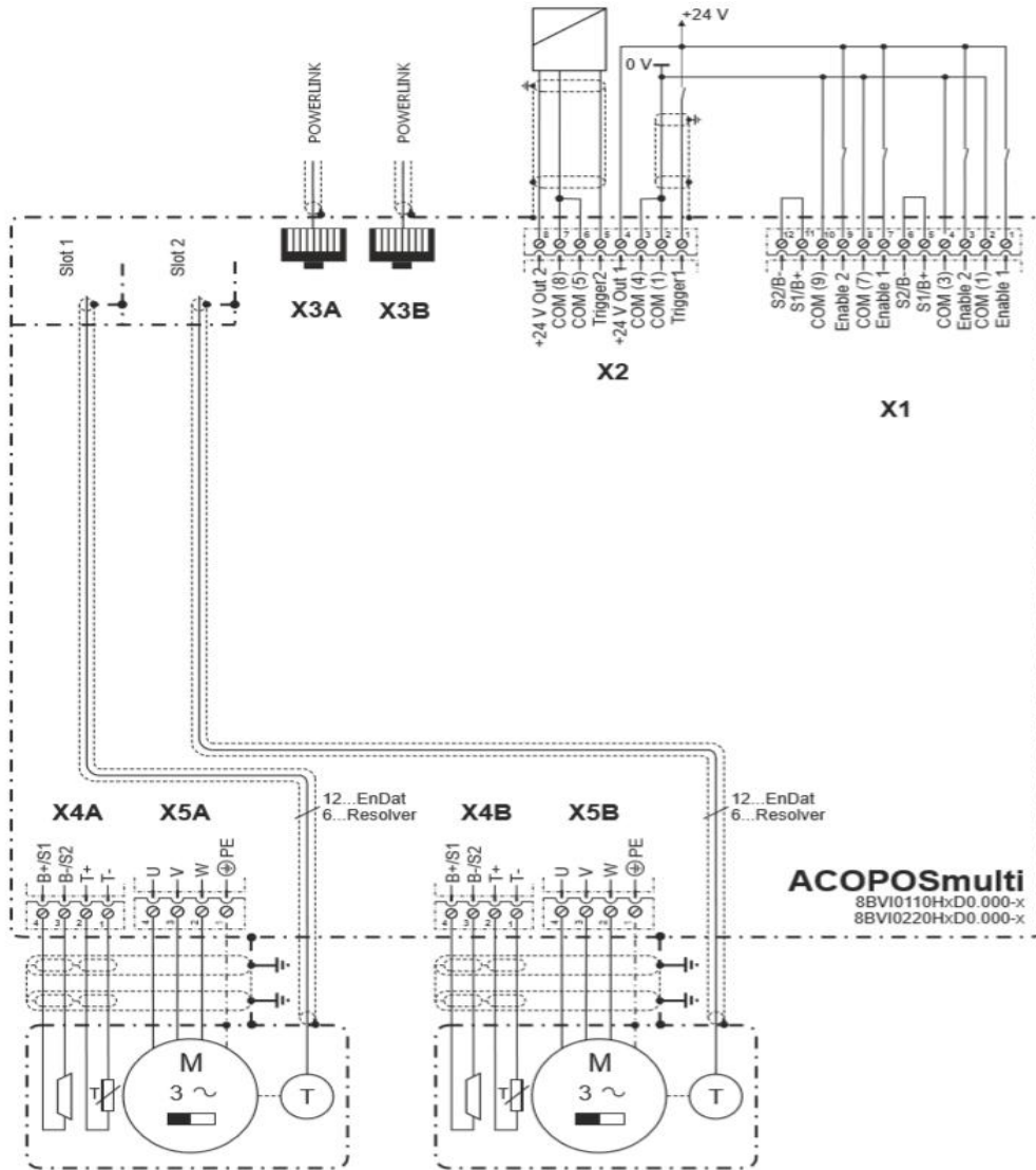
图 3-32 驱动器接线示意图
