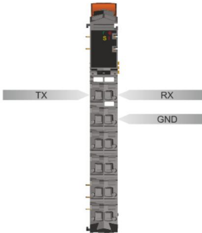
图 3-16 RS232 接口
