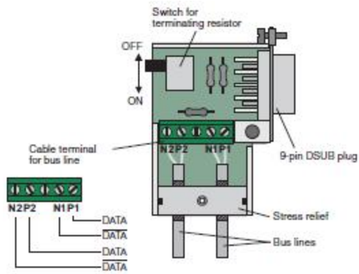
图 2-39 模块连接
