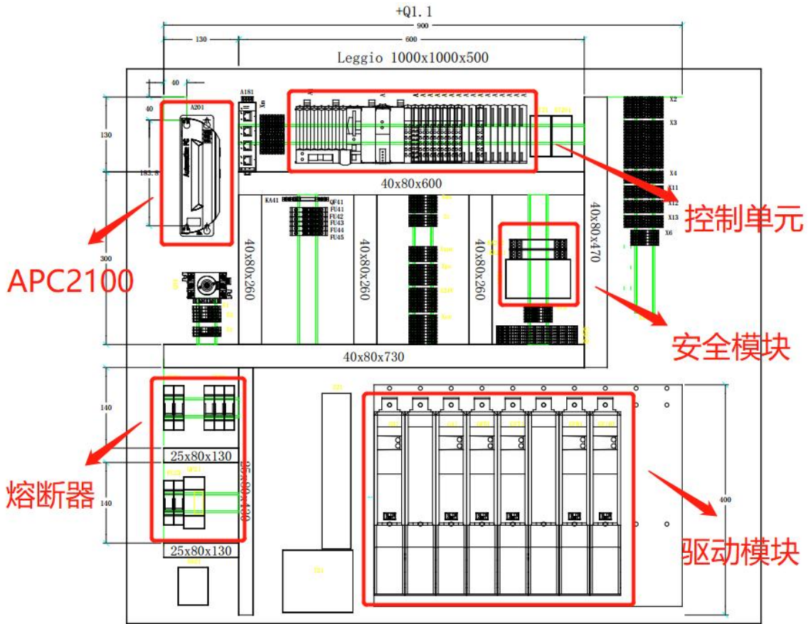
图 3-4 柜内布局图
