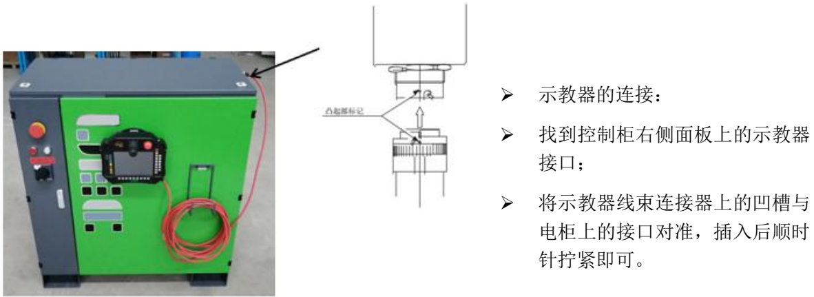
图 2-11 示教器的连接
