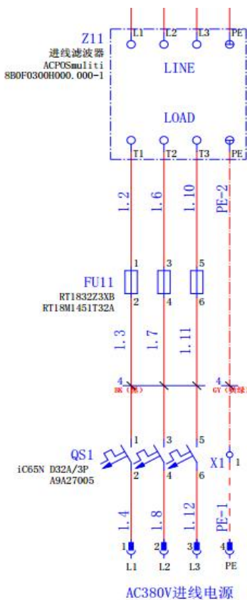
图 2-10 电源进线
