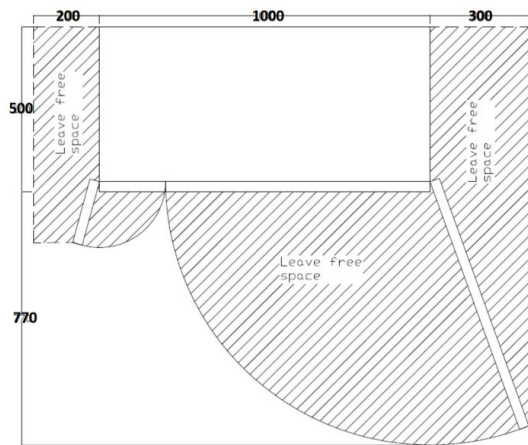
图 2-4 电控柜的安装要求
