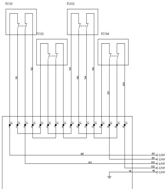
图 2-17 多个安全门连接接线图
