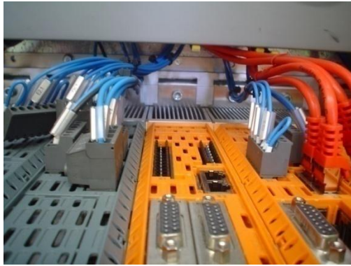
图 4-17 更换驱动器
