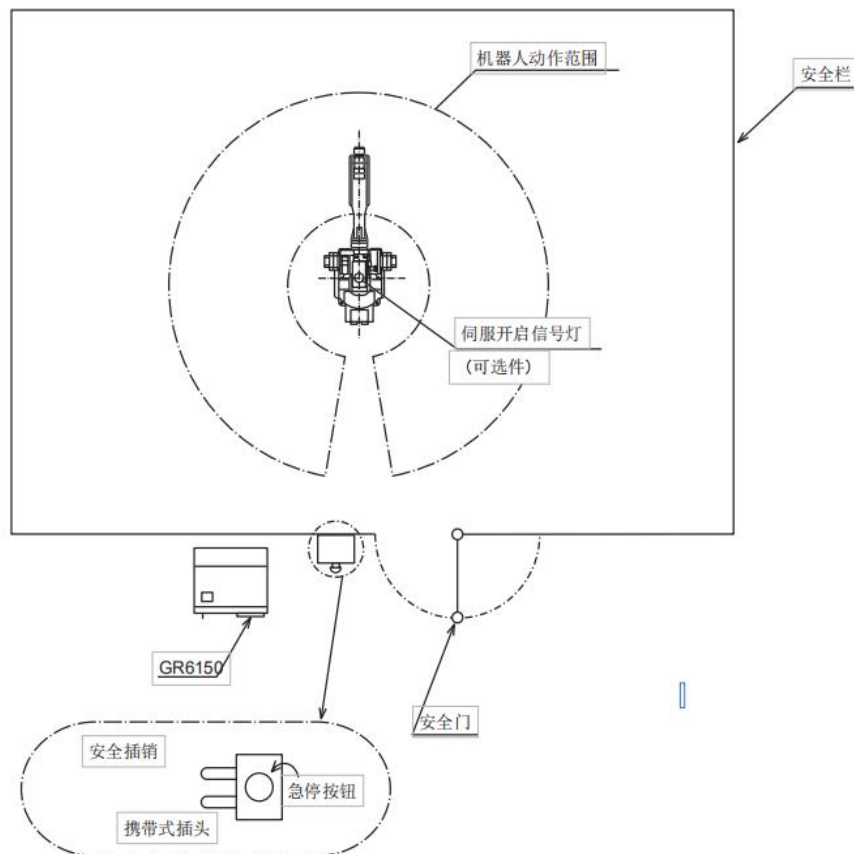
图 2-14 安全门应用实例
