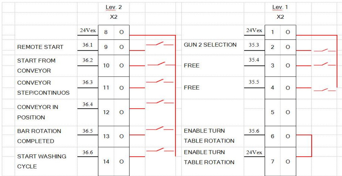
图 2-28 输入信号接线示意图
