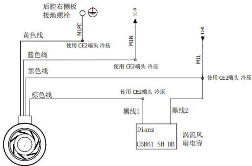
图 4-6 风扇
