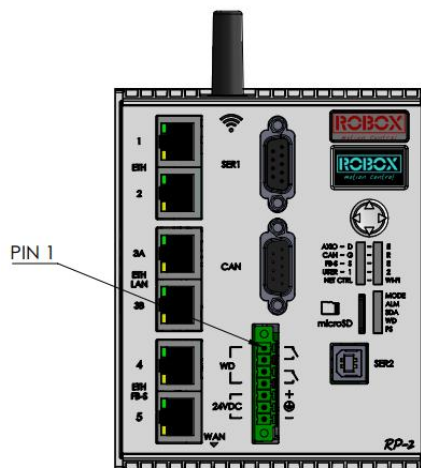
图 3-4 WD 端口位置指示图
