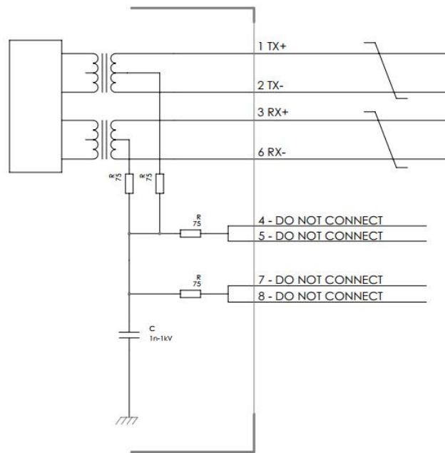
图 3-8 ETH 端口定义及连接电路图
