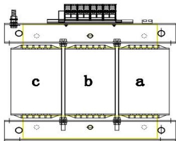
图 3-38 变压器
