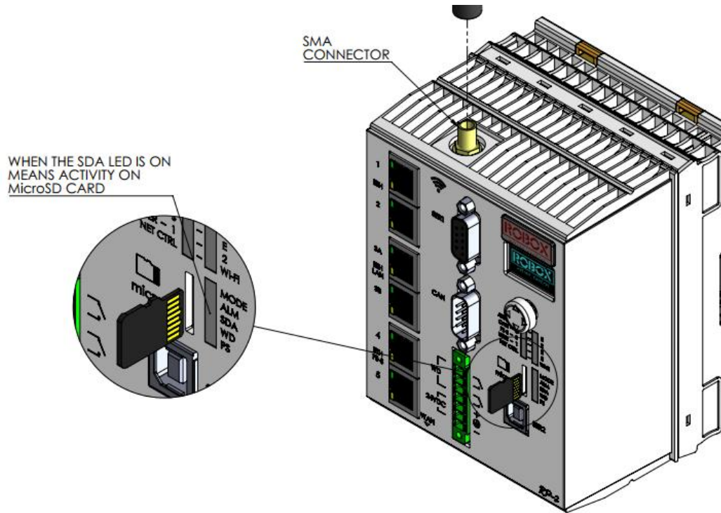
图 3-26 插入运动控制卡
