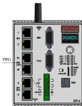
图 3-2 电源端口位置指示图
