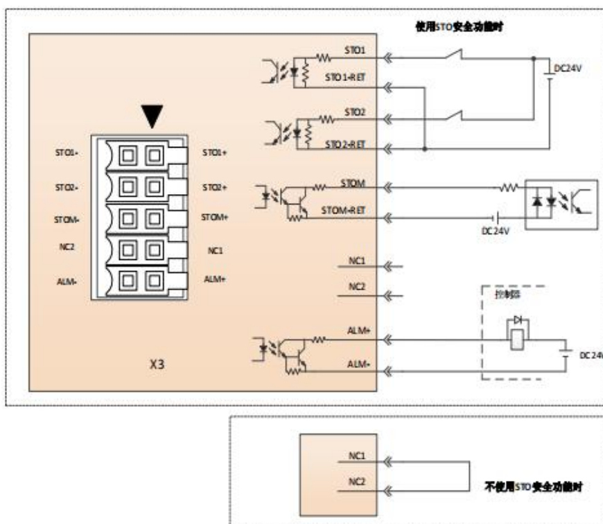
图 3-31 STO 接线图示
