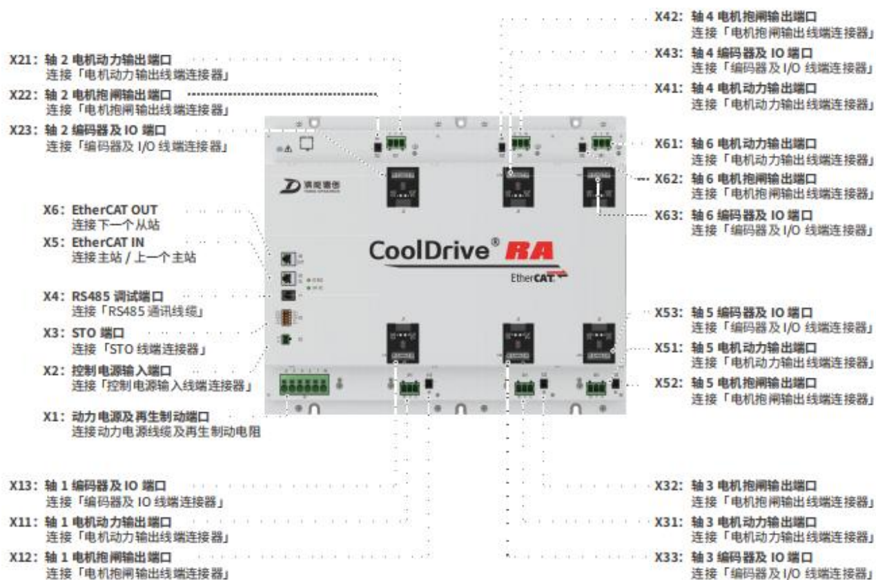
图 3-27 驱动器端口介绍
