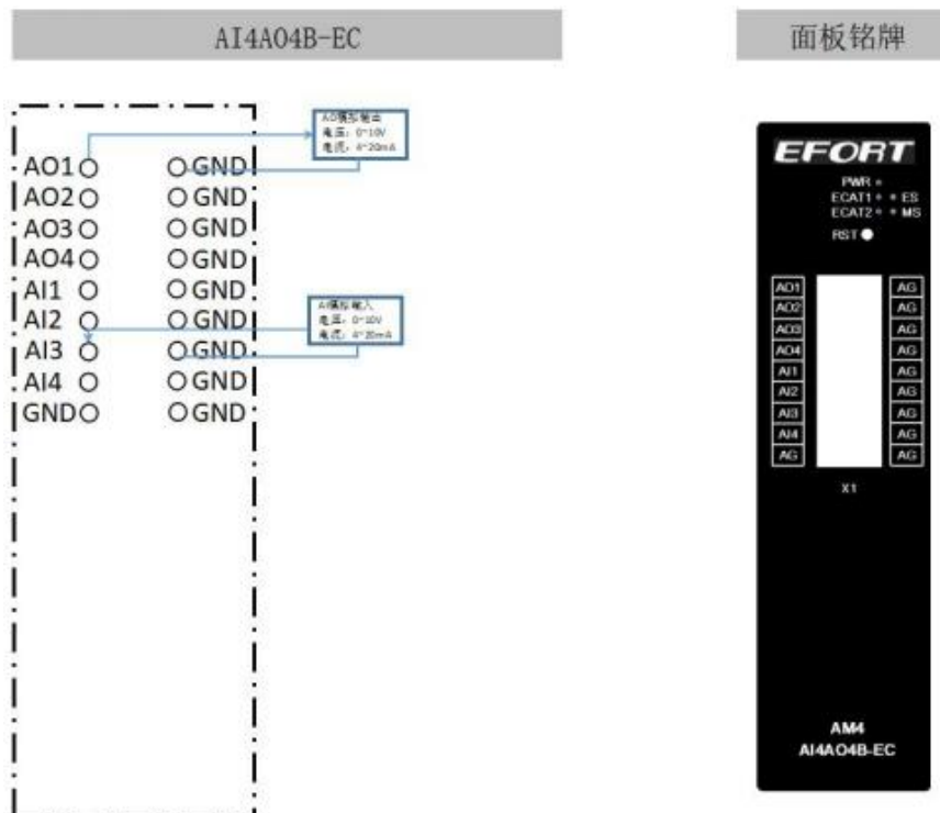
图 3-25 模拟量 I/O 接线方法示意图
