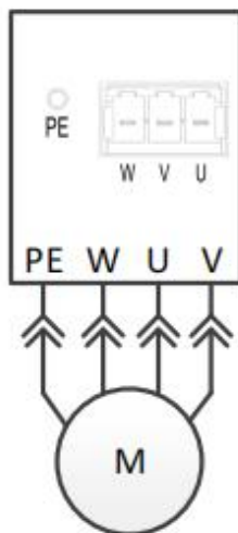
图 3-29 电机接线图示
