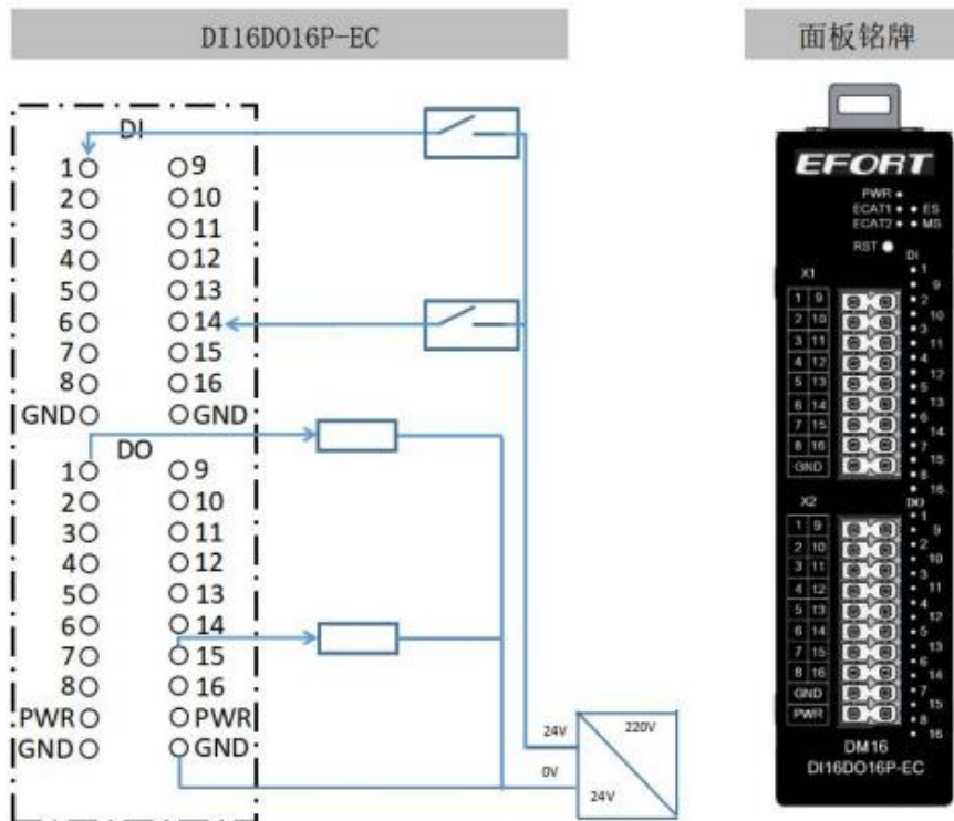
图 3-24 数字量 I/O 接线方法示意图
