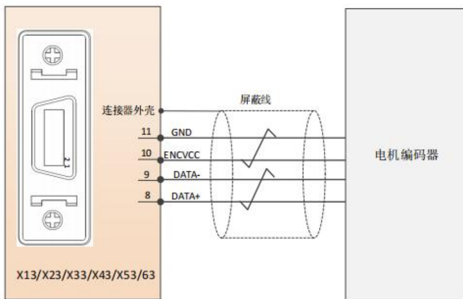
图 3-30 抱闸及编码器接线图示
