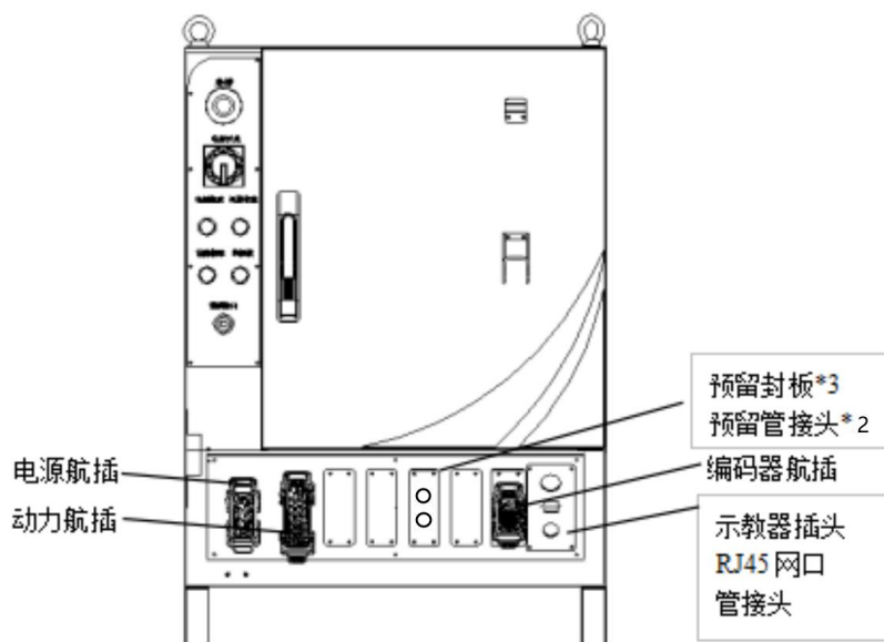
图 2-6 航插接口位置图
