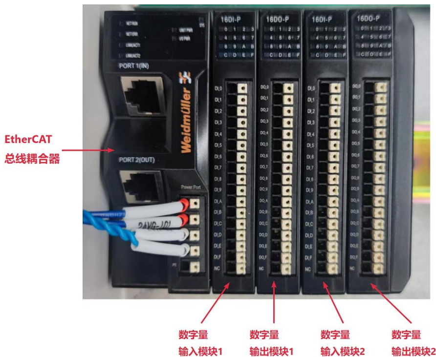
图 3-17 魏德米勒 IO 示意图
