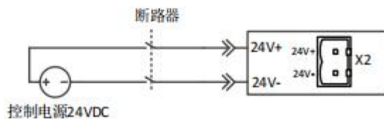
图 3-28 电源接线图示
