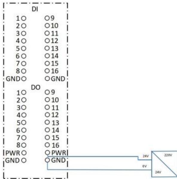
图 3-22 双电源接线方法示意图
