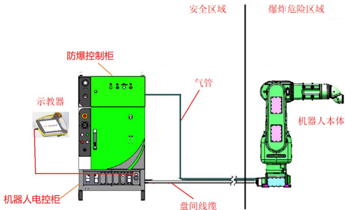
图 2-4 机器人线缆连接示意图
