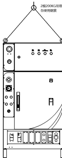
图 2-2 机器人控制柜吊装示意
