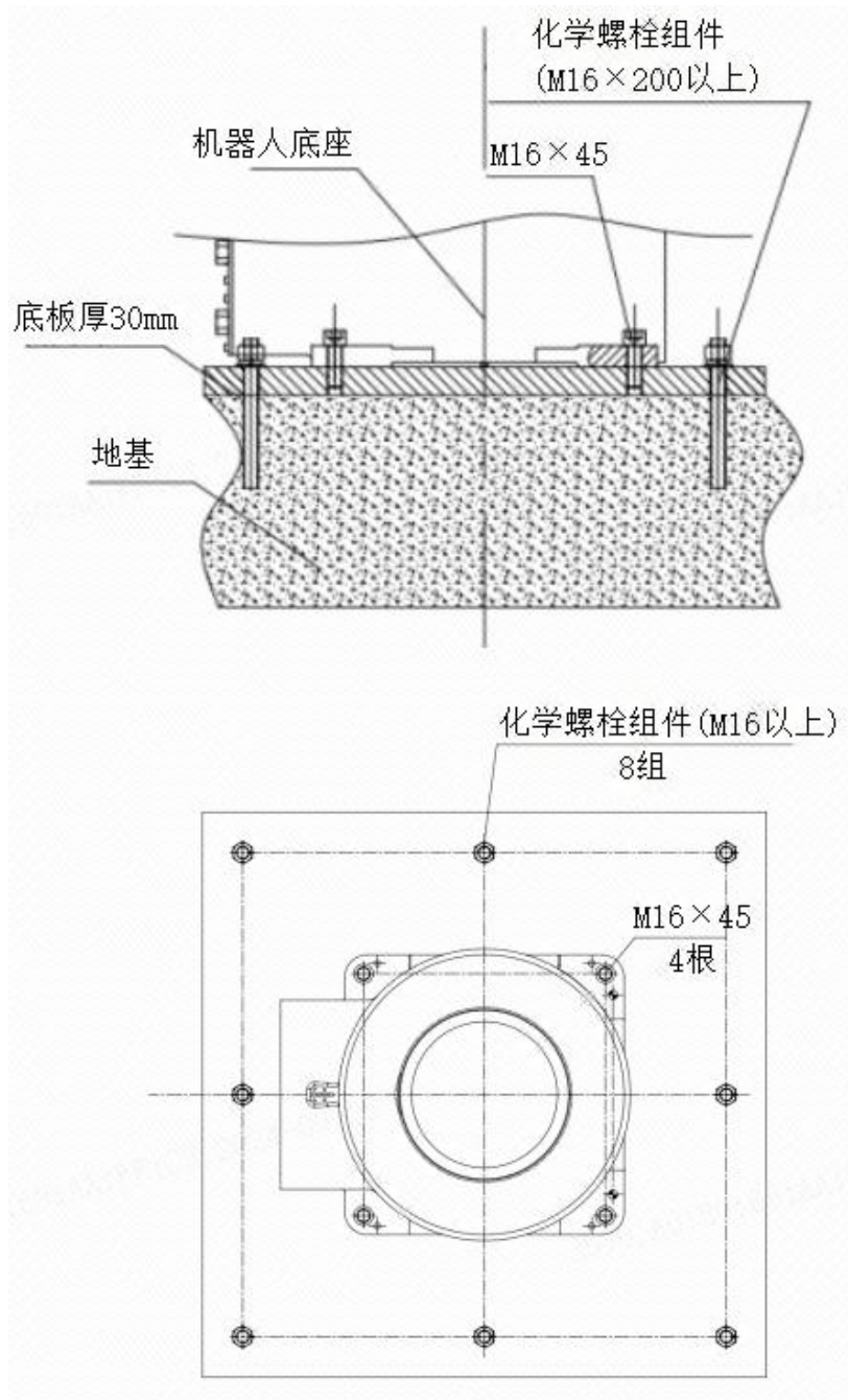
图 3-5 机器人安装举例
