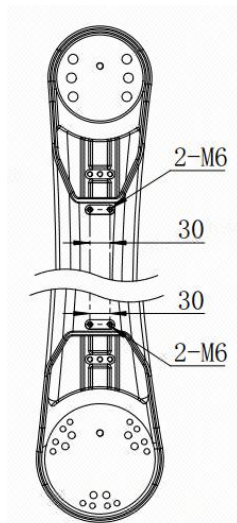
图 3-8 大臂上安装外部件尺寸图
