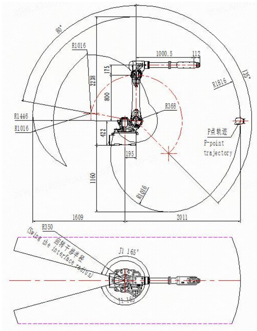
图 2-5 机器人工作空间图
