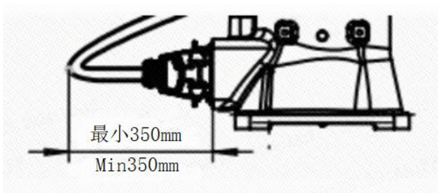
图 3-4 底座线缆后侧出线最小弯折尺寸
