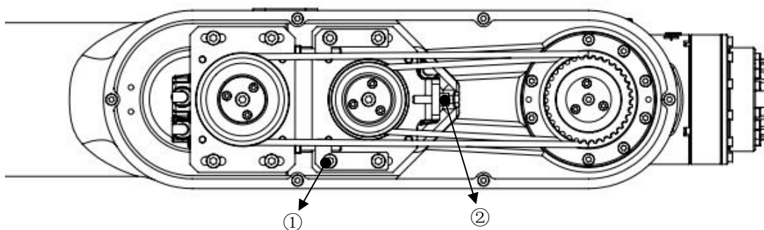
图 4-3 ER6-2000 机器人 J6 轴同步带结构图
