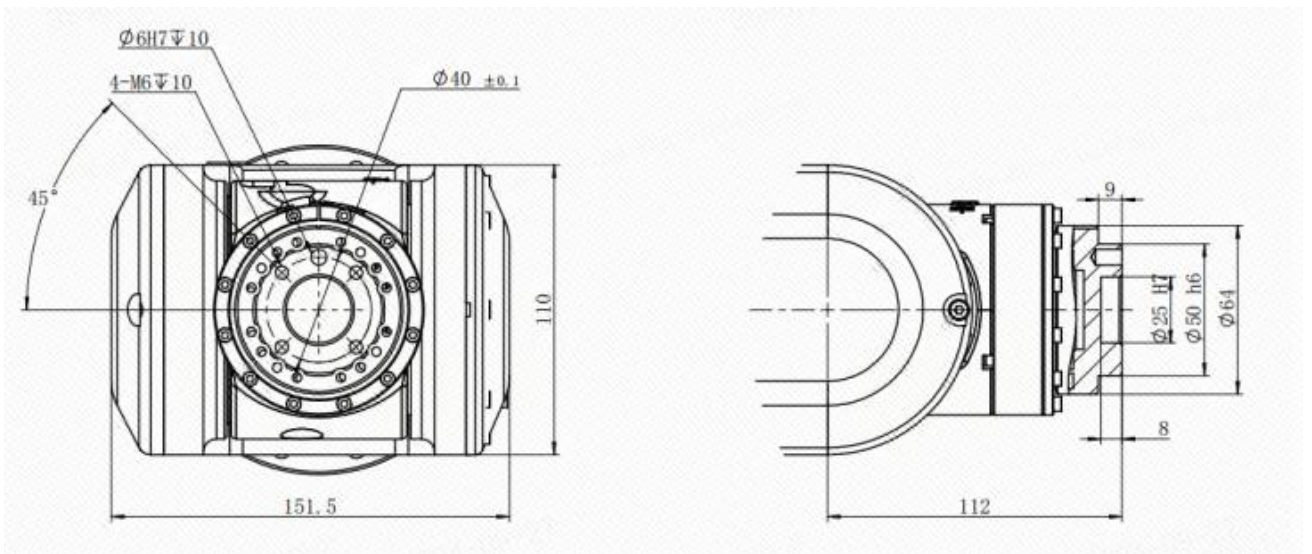
图 3-7 末端负载安装法兰尺寸
