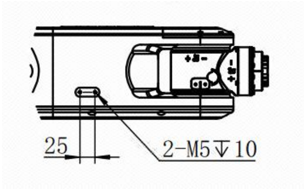
图 3-10 小臂杆上安装外部件尺寸图
