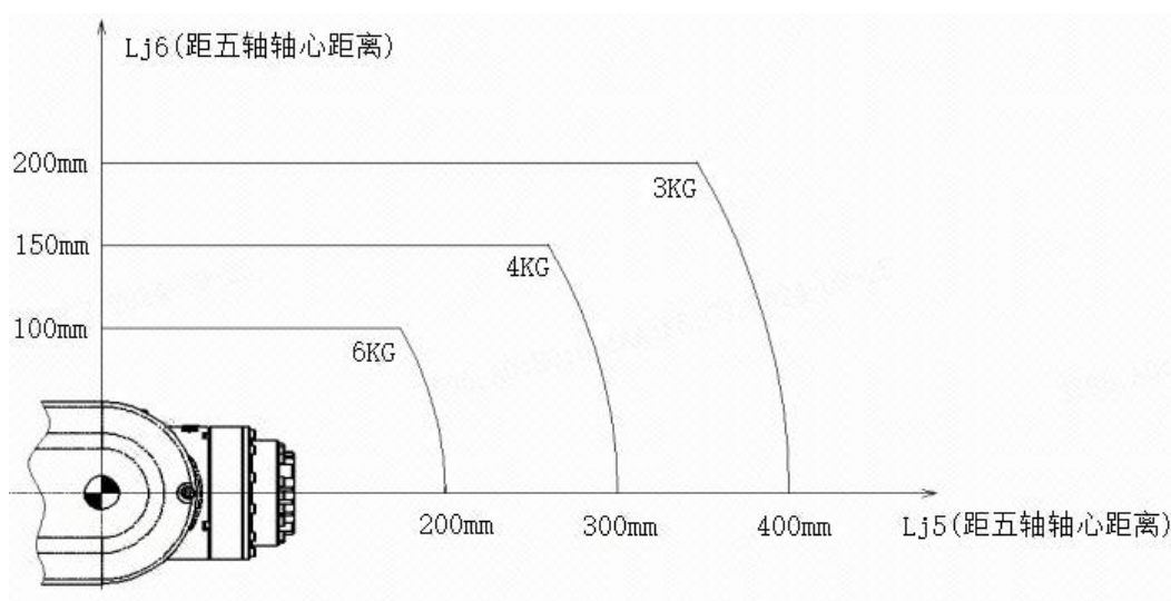
图 2-6 ER6-2000 手腕轴转矩图
