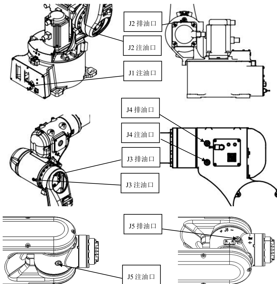
图 4-1 机器人注油口和排气口分布图
