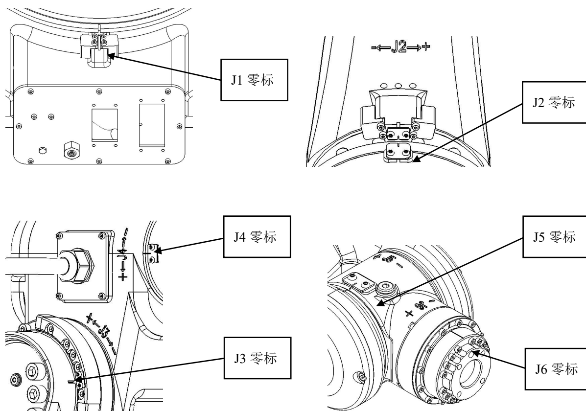
图 4-3 机器人零点位置图
