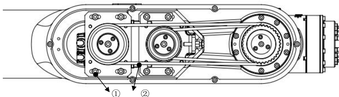
图 4-2 ER6-2000 机器人 J5 轴同步带结构图
