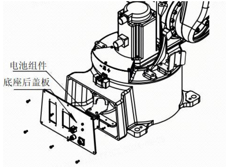
图 4-4 机器人电池组位置图
