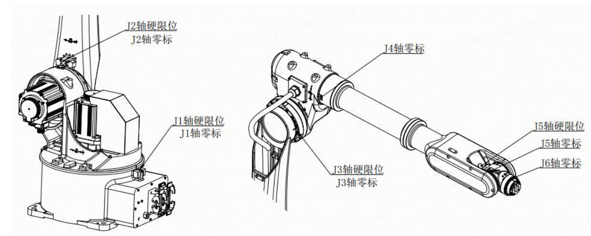
图 2-4 机械硬限位位置及零标位置
