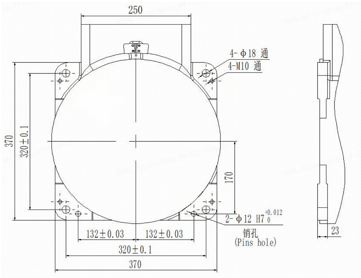
图 3-3 机器人底座尺寸
