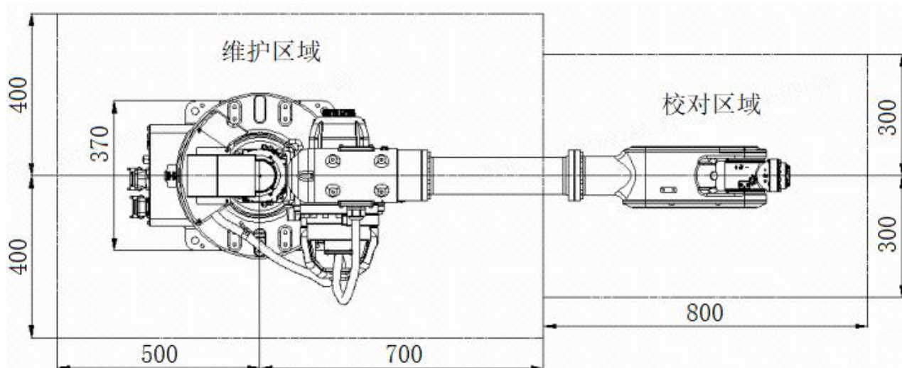
图 4-2 维护及使用区域
