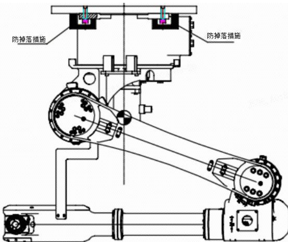
图 3-6 倒挂安装
