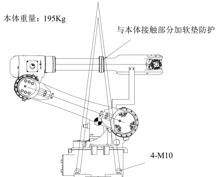
图 3-1 吊装搬运示意图
