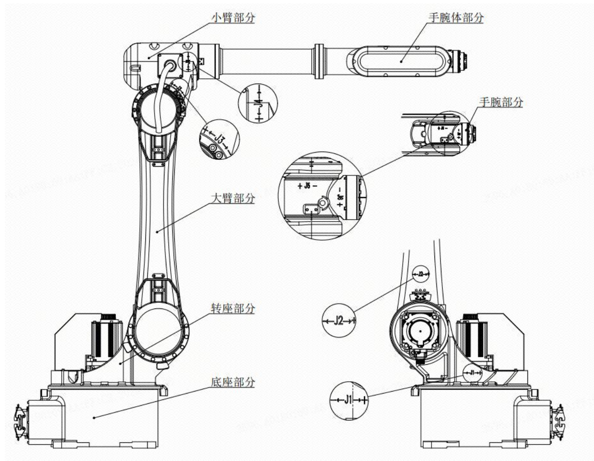
图 2-3 ER6-2000 机械本体组成部分
