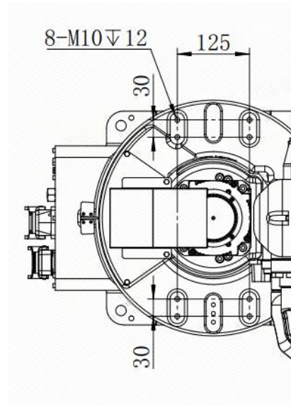
图 3-11 转座上安装外部件尺寸图
