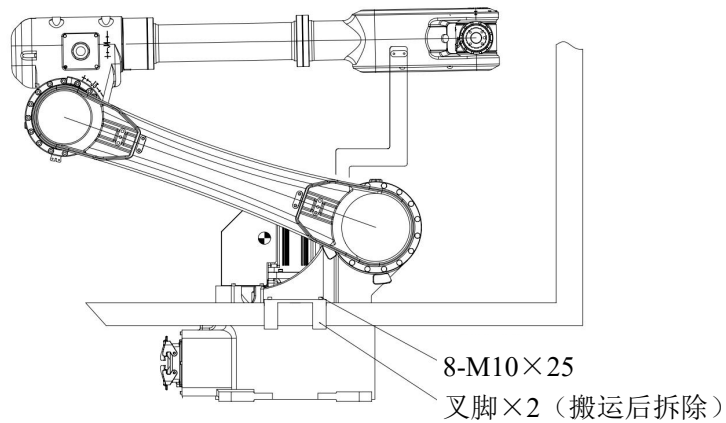
图 3-2 叉车搬运示意图
