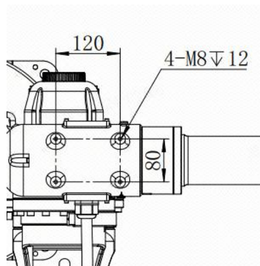
图 3-9 电机座上安装外部件尺寸图
