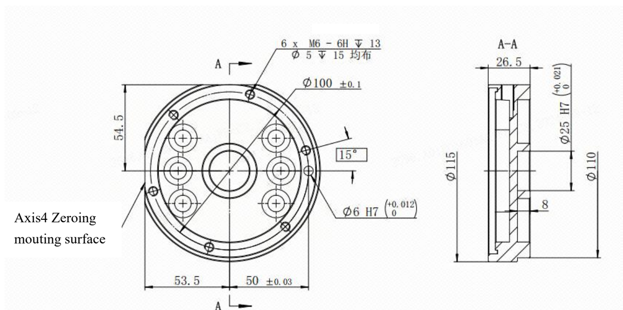
图 3-9 末端负载安装法兰尺寸图
