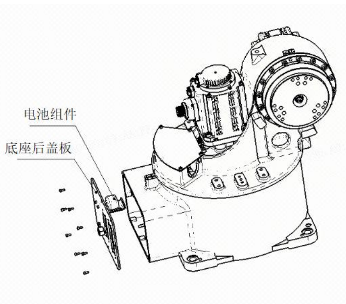
图 4-4 机器人电池组位置图
