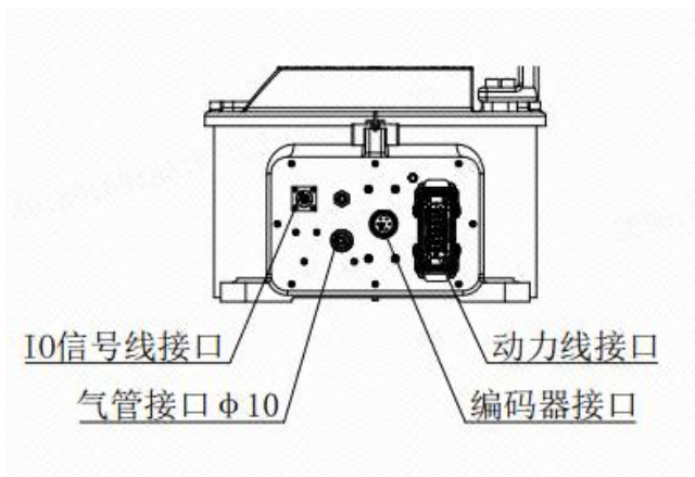
图 3-13 底座部分气路及信号线接口
