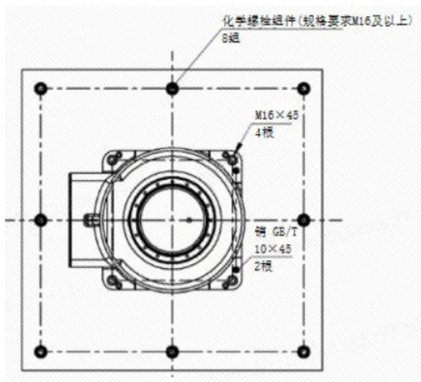
图 3-7 机器人安装举例
