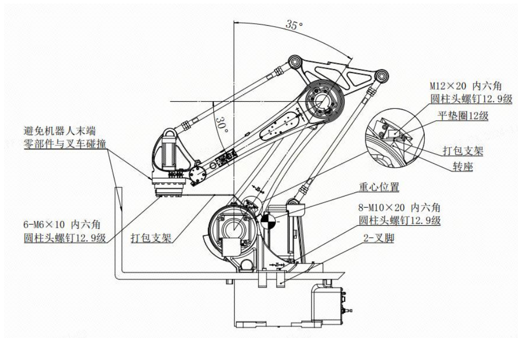
图 3-4 叉车搬运示意图
